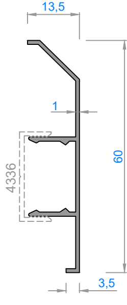
3918 - 0,272 kg/m
