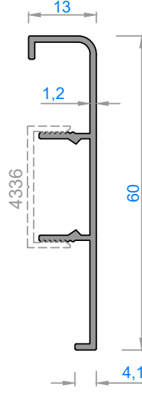
4830 - 0,320 kg/m
