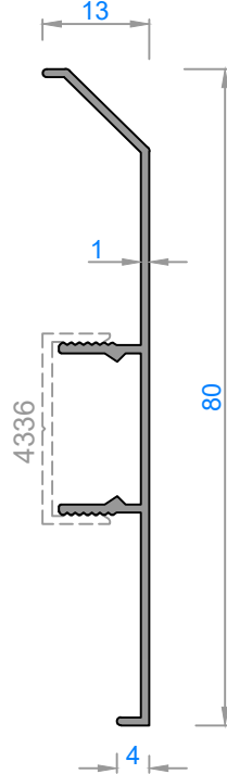
4346 - 0,313 kg/m
