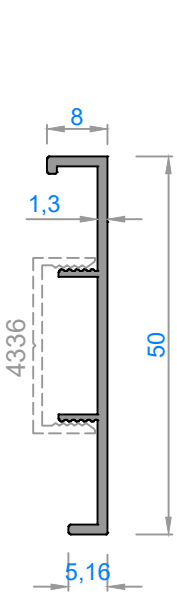
5434 - 0,245 kg/m
