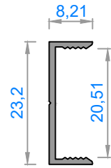
4336 - 0,120 kg/m
