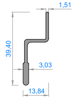
1142 - 0,407 kg/m
