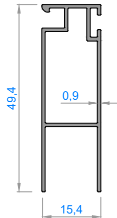
4700 - 0,344 kg/m
