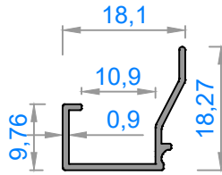
1990 - 0,111 kg/m
