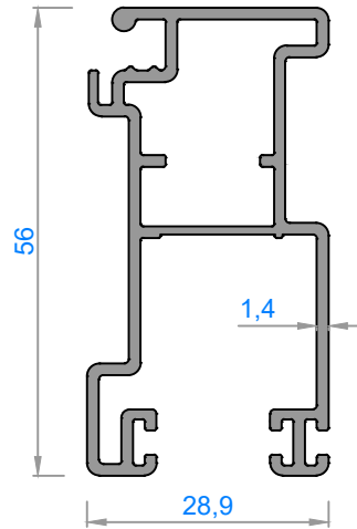
4731 - 0,800 kg/m
