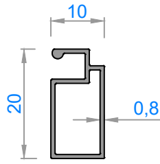
1727 - 0,143 kg/m
