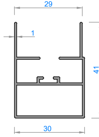
4252 - 0,453 kg/m
